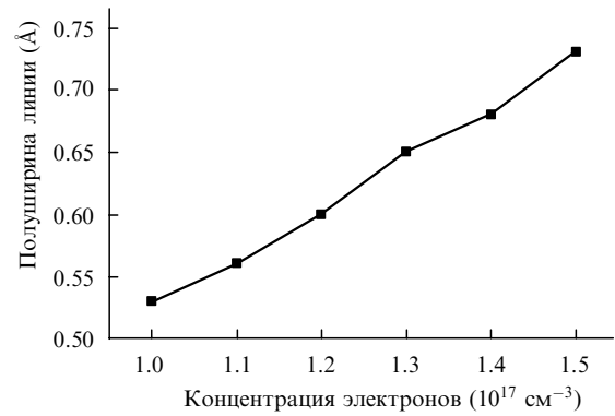
Рис.2. Зависимости полуширины спектральной линии первого иона углерода С II с \lambda = 392.0 нм от концентрации электронов.
