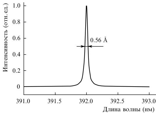
Рис.1. Профиль линии первого иона углерода С II с \lambda = 392.0 нм при T = 1.82 эВ и N_e = 1.12 \times 10^{17} см ^{-3} .
