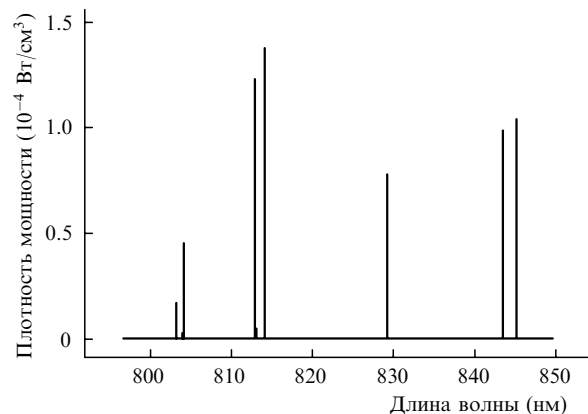
Рис.6. Неравновесный спектр плазмы аргона, полученный при T_e = 0.95 эВ, T_i = 0.73 эВ, N_e = 8.5 \times 10^{13} см ^{-3} .
