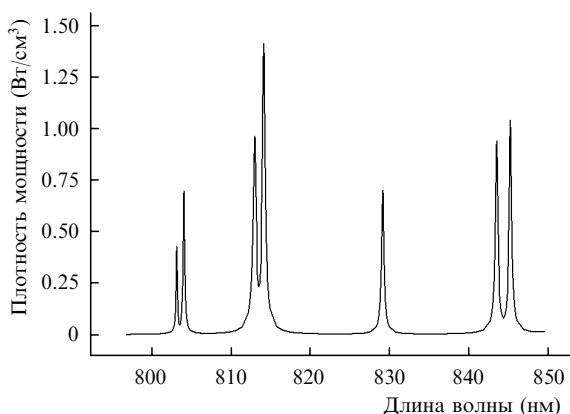
Рис.9. Равноесный спектр плазмы аргона, полученный при T = 2.35 эВ, и N_e = 1.8 \times 10^{17} см ^{-3} .
