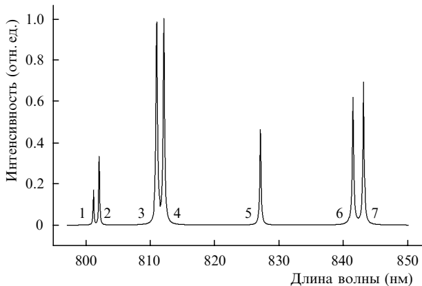
Рис.3. Равновесный спектр излучения плазмы аргона, вычисленный при T = 2.2 эВ, N_e = 1.1 \times 10^{17} см -3 .
