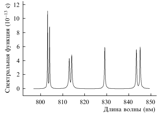
Рис.10. Спектральная функция S(\lambda) , соответствующая равносному спектру на рис.9.
